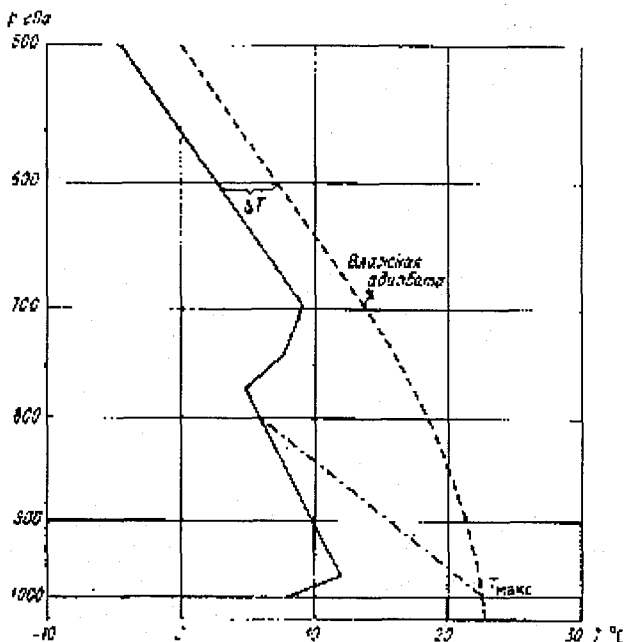
Рис. 7.6. График для прогноза максимальных порывов ветра у земли при грозах.
