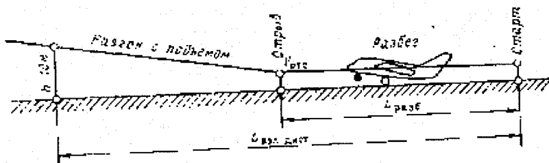
Рис. 3.4. Этапы взлета самолета.
