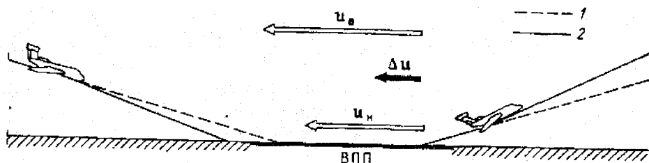
Рис. 7.3. Пример влияния вертикального сдвига ветра на взлет и посадку:
