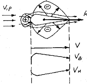
Рис. 1.3. Обтекание крыла потоком при \alpha = 0 .
