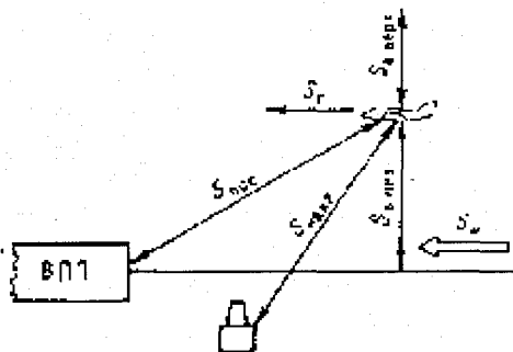
Рис. 9.2. Характеристики видимости, используемые при метеорологическом обеспечении полетов.
