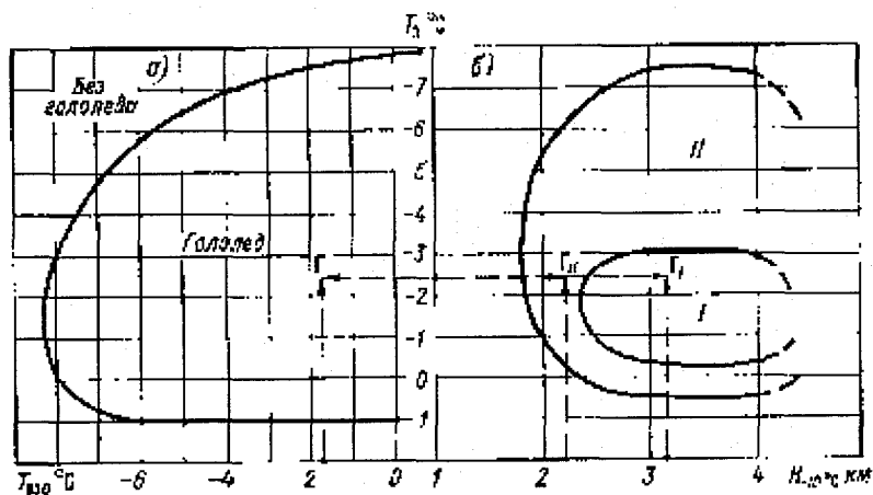
Рис. 10.3. Номограмма Р.А. Ягудина для определения возможности возникновения гололеда (а) и его интенсивности (б): I – зона умеренного гололеда; II – зона слабого гололеда.
