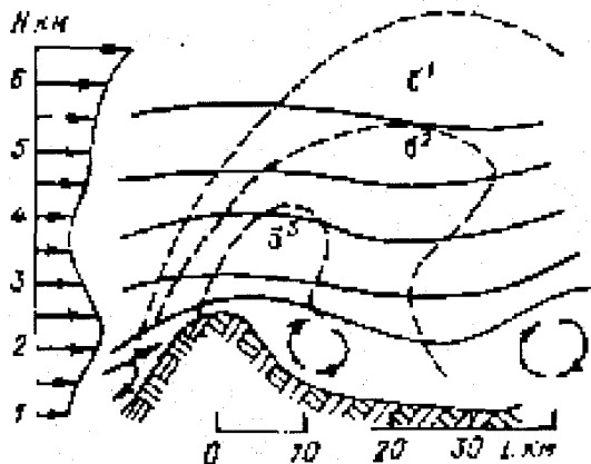
Рис. 8.5. Характеристика турбулентных зон над горами. \text{б}^1 – слабая, \text{б}^2 – умеренная, \text{б}^3 – сильная болтанка.
