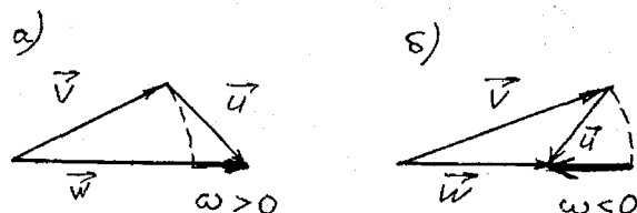
Рис. 7.2. К определению эквивалентного ветра: a - \omega > 0, б - \omega < 0 .
