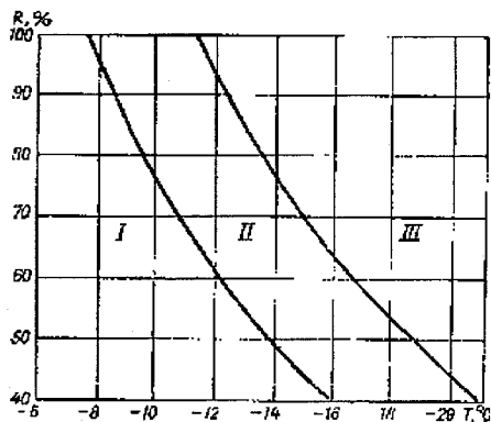
Рис. 9.24. График для прогноза туманов испарения.
