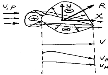
Рис. 1.4. Обтекание крыла потоком при \alpha > 0 .
