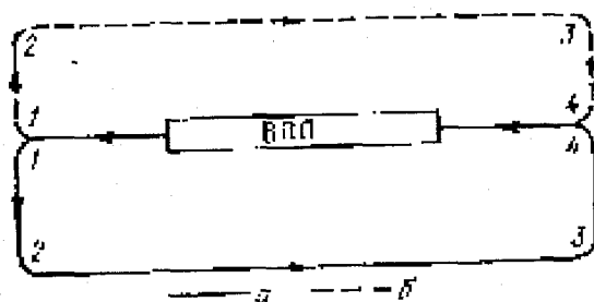
Рис. 5.1. Схема круга над аэродромом: а – левый круг, б – правый круг; 1, 2, 3, 4 – места первого, второго, третьего и четвертого разворотов соответственно.
