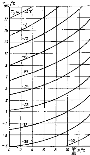
Рис. 11.2. График для определения температуры нулевого испарения.
