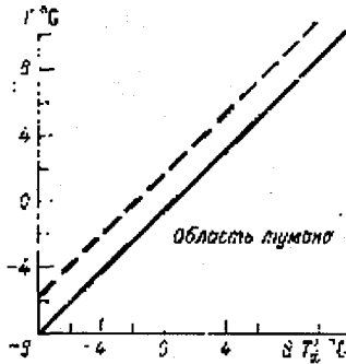
Рис. 9.23. График для прогноза адвективного тумана (по методу А.А. Шадринной).
