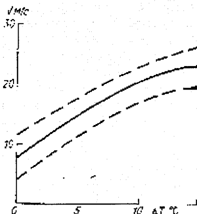
Рис. 7.15. График для определения скорости ветра при шквале, используемый в Новосибирске.
